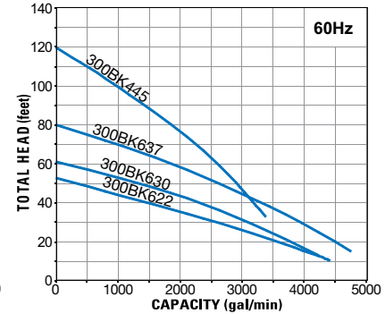
Discharge Size: 12"
